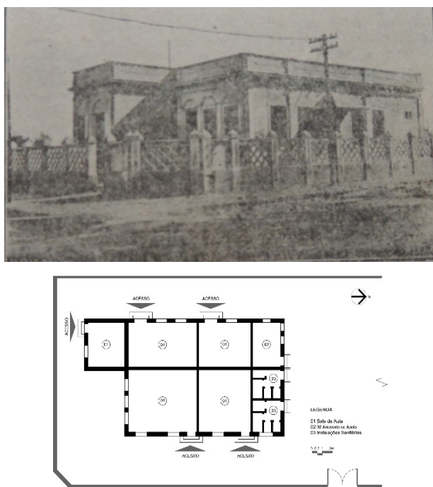
Figuras 3 e 4 – Fotografia do Mariana Eufrásia (1924). Planta baixa do Mariana Eufrásia
